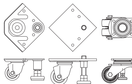
SCY-250/350
